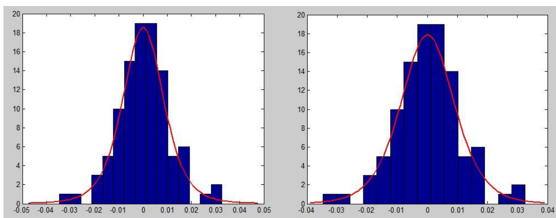
图 3.2 对实际收益率进行 t 分布拟合
